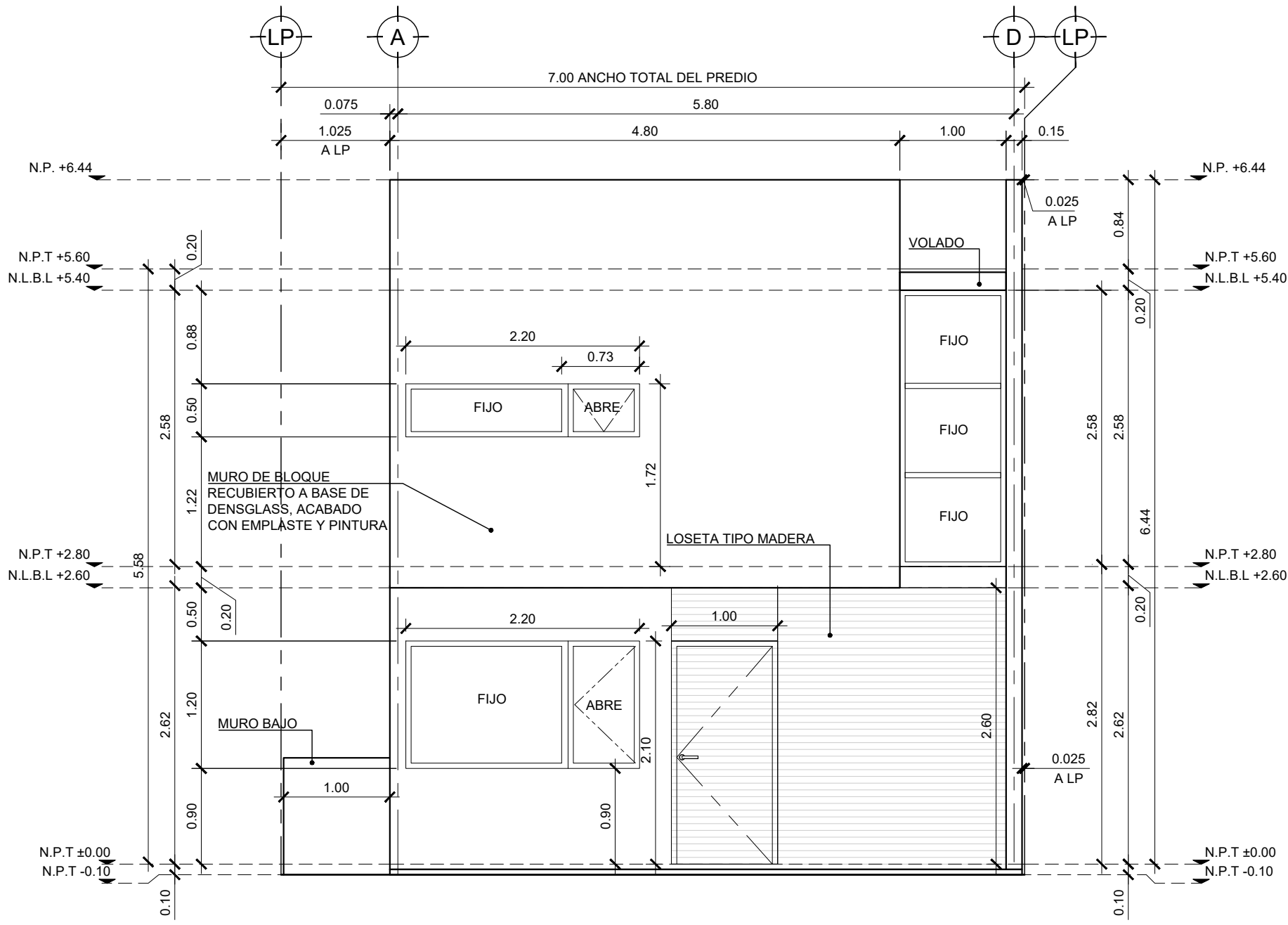
FACHADA FRONTAL ESC 1:50
