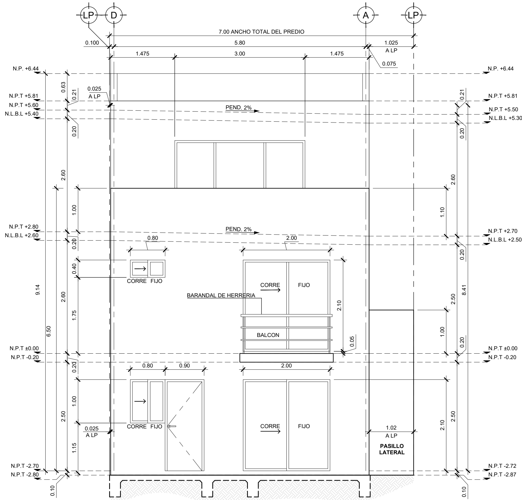
FACHADA TRASERA ESC 1:50
